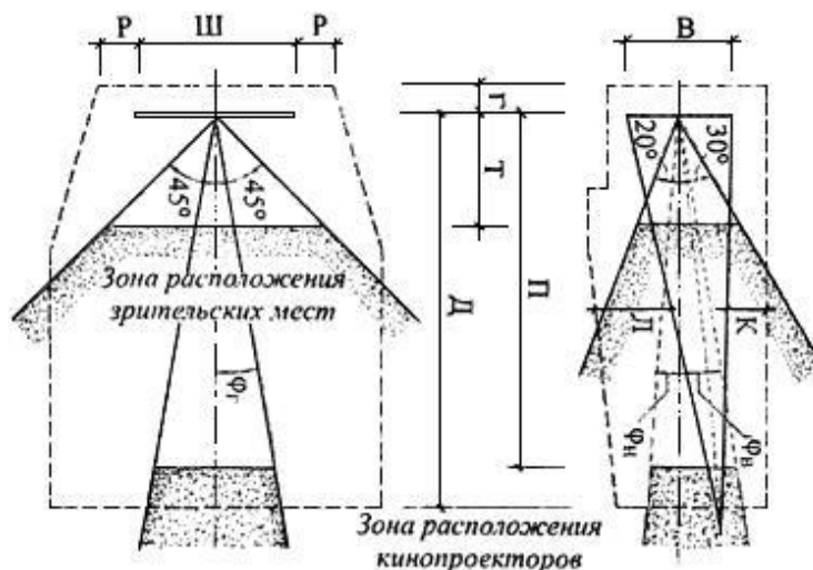
Рисунок Е.1 - Параметры зрительного зала и киноэкрана при кинодемонстрации в залах кинотеатров и универсальных залах
