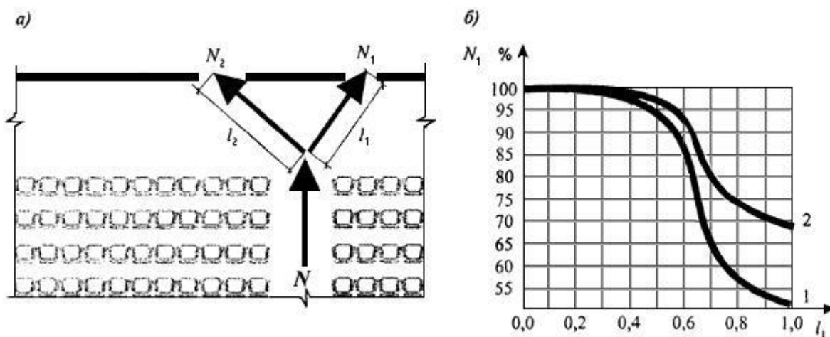
Рисунок И.3 - Распределение численности зрителей между выходами
