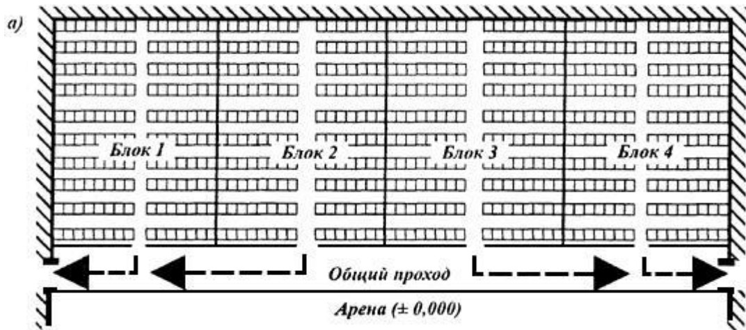
Рисунок И.2 - Схемы разделения мест на блоки на трибунах спортивно-зрелищных и универсальных залов при расположении люков
